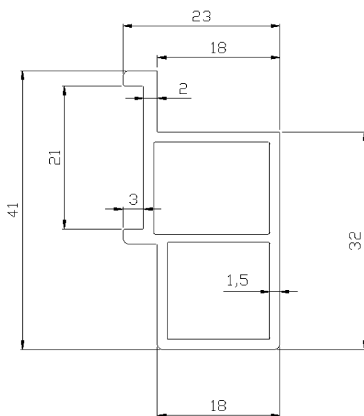
Figura 1 Profilo telaio pianale
