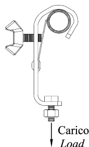
Figura 1 Configurazione di lavoro.
